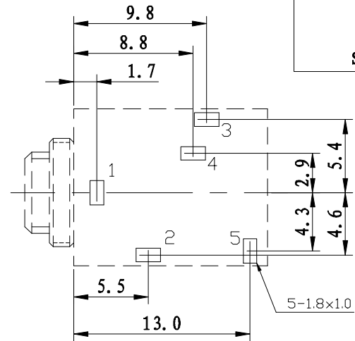
线路板安装尺寸示意图
