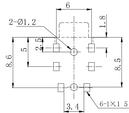
PCB 板开孔尺寸
