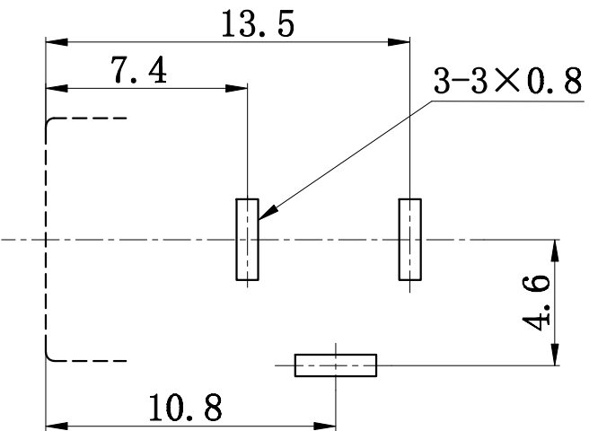
线路板开孔尺寸
